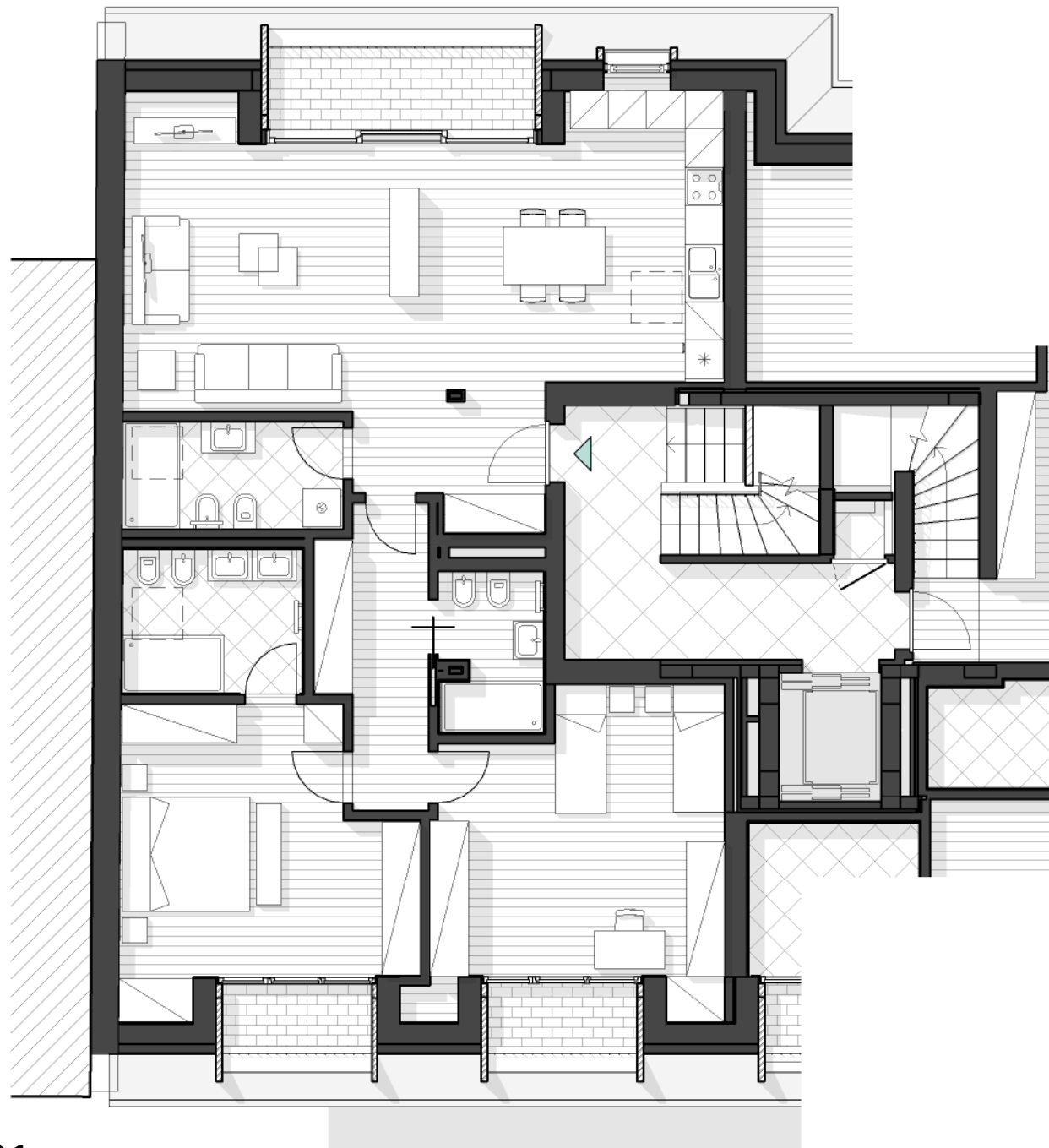
6.01 Unità al 6° piano Einheit im 6. Obergeschoss
